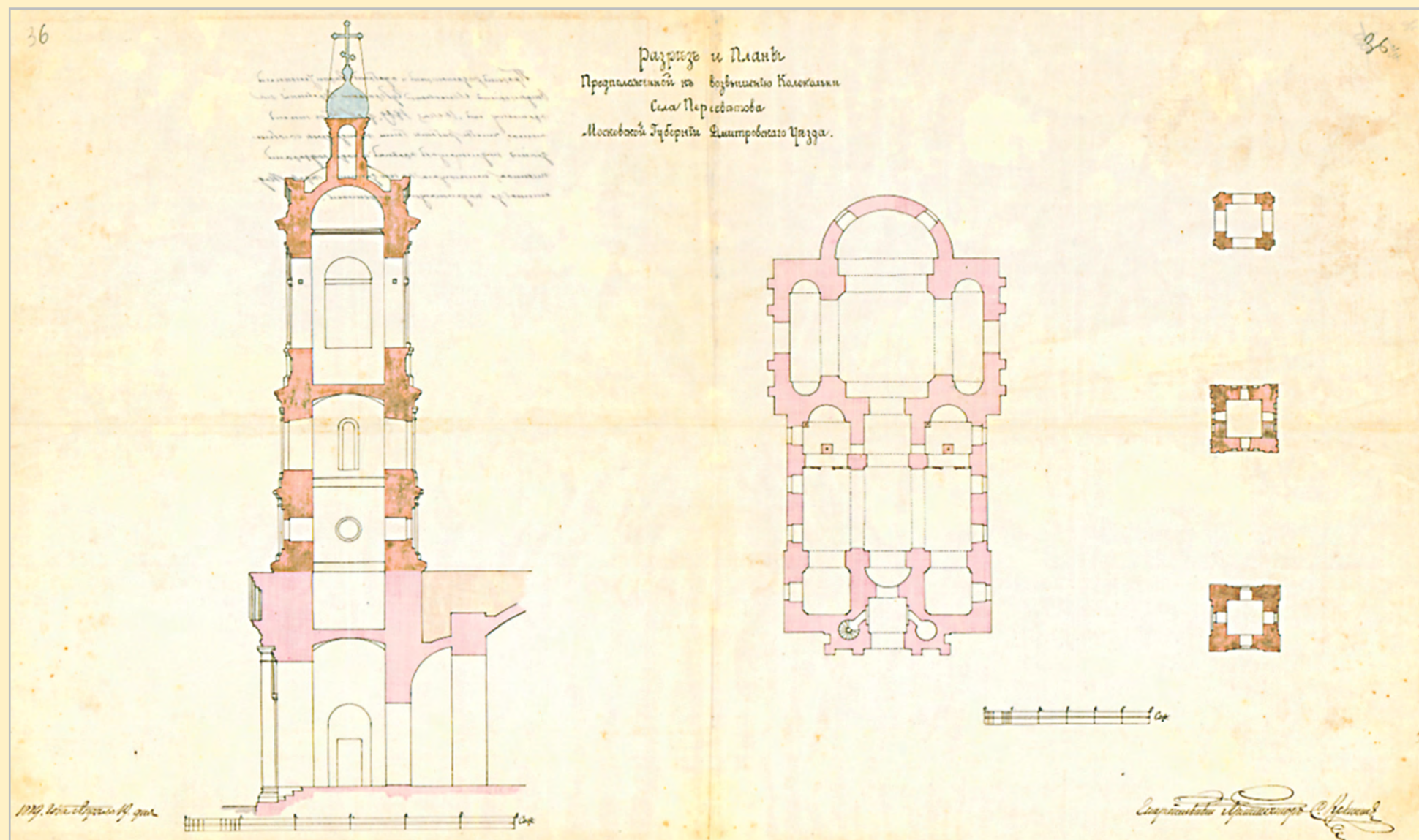
Разрез и планы Скорбященской церкви села Пересветово с колокольней. 1889 год. Архитектор С.В. Крыгин
